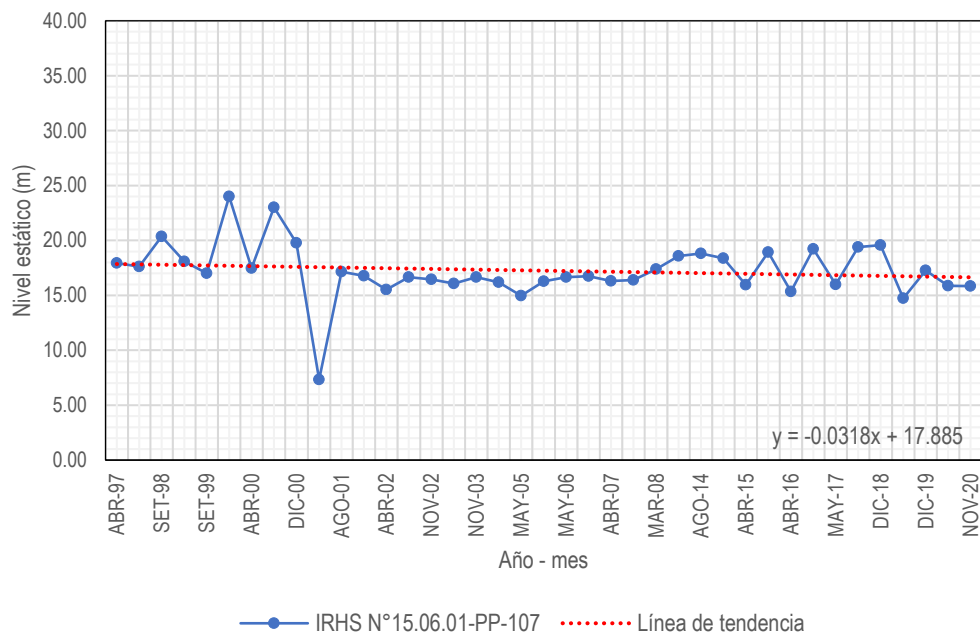
HIDROGRAMA IRHS N°15.06.01-PP-107
