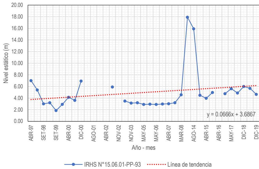
HIDROGRAMA IRHS N°15.06.01-PP-93
