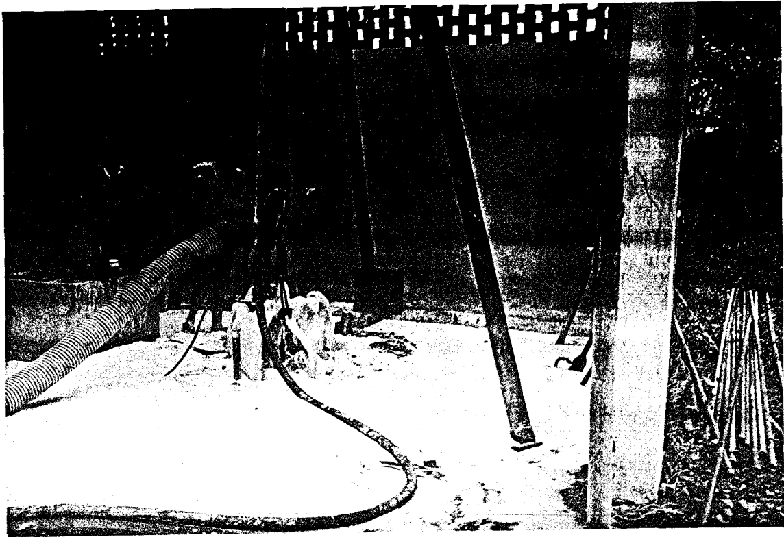
Fig. 03 Realizando rebose del pozo se nota el aditivo químico
