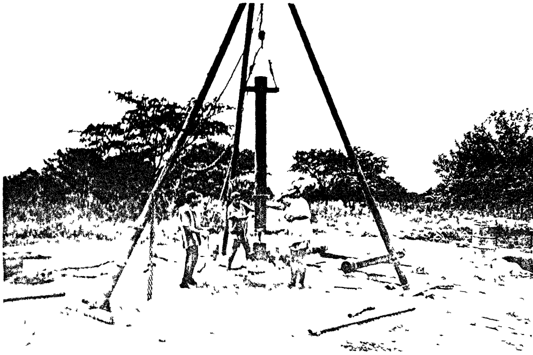
Fig. 03 Instalación de equipo de prueba
