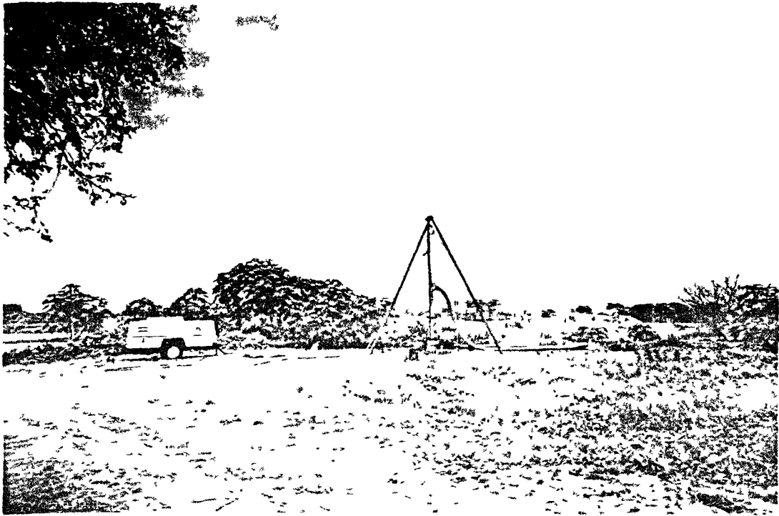
Fig. 01 Limpieza y recuperación de fondo con aire comprimido
