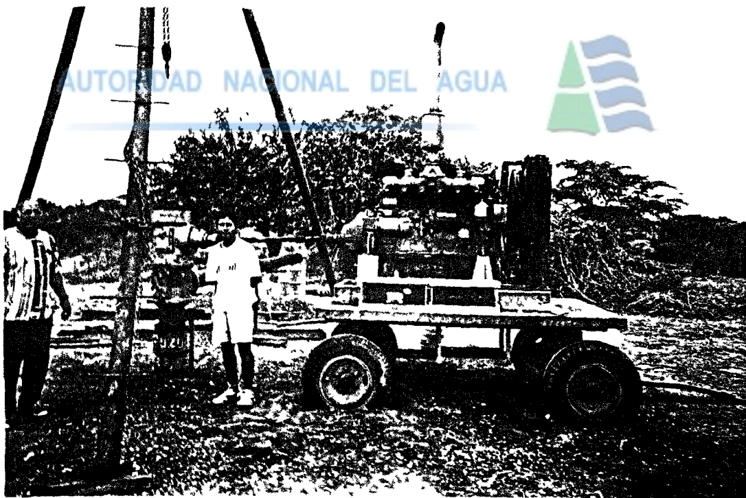
Fig. 04 Equipo de prueba de rendimiento instalado
